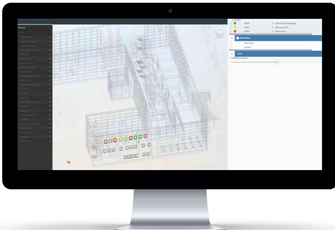
Abbildung 18: Nachverfolgung von Instandhaltungs- und Instandsetzungsmaßnahmen auf Basis eines Bauwerksinformationsmodells
